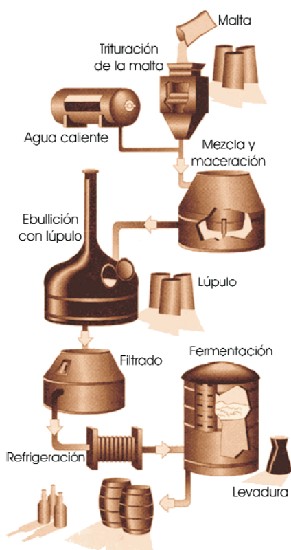
Ilustración 9.25. Proceso de fabricación de la cerveza tipo Ale por fermentación alta; es decir, la fermentación de la malta, realizada por la levadura Saccharomyces cerevisiae , se produce en la superficie exterior (Fuente: http://www.bolsonweb.com ).
