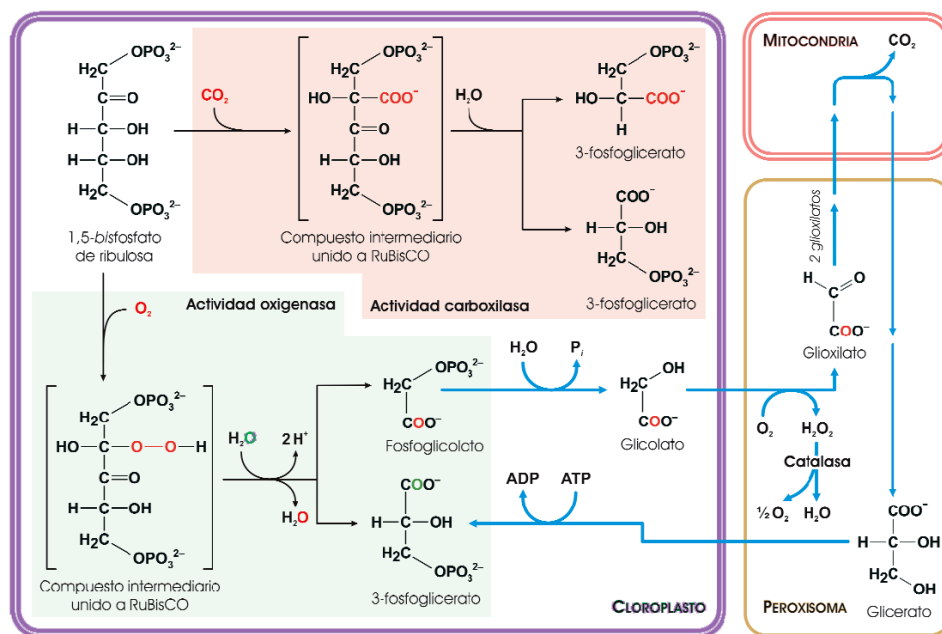
Ilustración 9.10. La fotorrespiración de las plantas (flechas gruesas de color azul celeste) se debe a que RuBisCO, además de su actividad como carboxilasa, posee también actividad como oxigenasa (Fuente: ASH).
