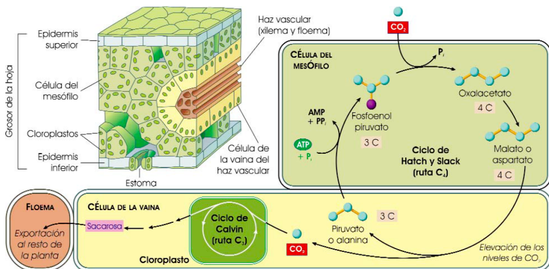
Ilustración 9.11. Corte transversal de la hoja de una planta con la ruta \text{C}_4 . Las células del mesófilo, próximas a los espacios aéreos de la hoja, fijan el \text{CO}_2 y lo bombean a las células que rodean el tejido vascular, donde se localiza RuBisCO (Fuente: ASH).
