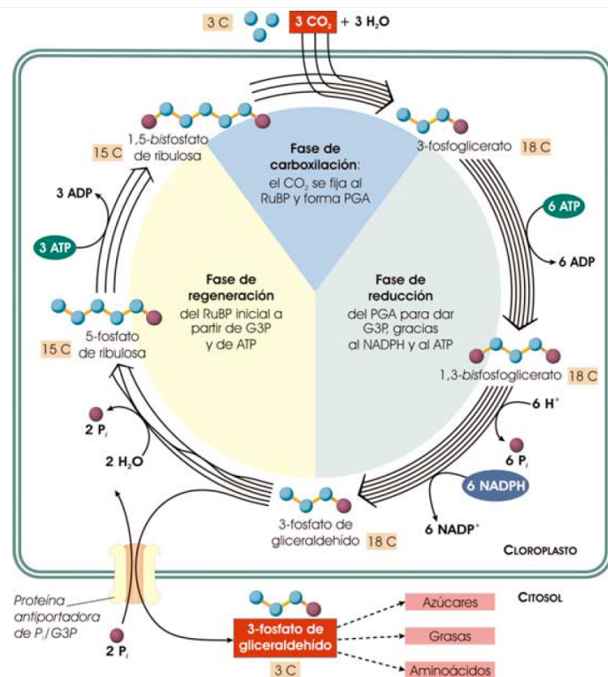
Ilustración 9.9. En el curso de tres vueltas del ciclo de Calvin se fijan tres moléculas de CO 2 a otras tantas de RuBP, formándose, tras una fase reductora, seis moléculas de G3P (las seis líneas de la flecha); cinco de ellas experimentan una serie de reacciones que regeneran las tres moléculas de RuBP iniciales, lo que deja como “ganancia” neta una molécula de G3P (Fuente: ASH).
