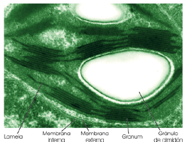
Ilustración 9.15. Izquierda: esquema de la estructura de un cloroplasto. Derecha: fotografía tomada con el MET del meristemo apical del cóleo ( Coleus blumei ), mostrando un cloroplasto (Fuentes: http://es.wikipedia.org/wiki y http://remf.dartmouth.edu ).
