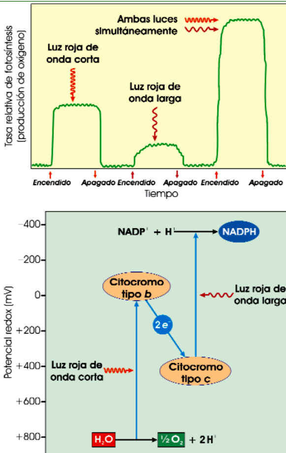
Ilustración 9.12. El efecto Emerson (arriba) y su interpretación según Hill y Bendall (abajo). (Fuente: ASH).
