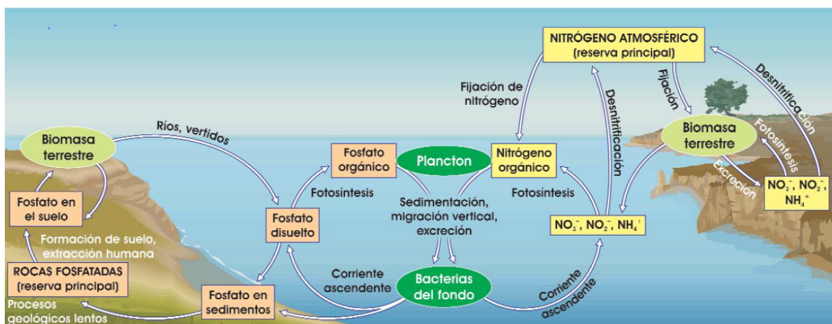
Ilustración 9.24. Representación conjunta de los ciclos del nitrógeno y del fósforo. Obsérvese que, aunque el reservorio natural del nitrógeno es la atmósfera, este elemento solo puede ser fijado por algunos seres vivos y además su fijación es muy costosa energéticamente, por lo que a menudo es un factor limitante para el crecimiento y desarrollo de los seres vivos. En cuanto al fósforo , este elemento no se presenta en estado gaseoso en condiciones de temperatura y presión normales. Su ciclo se realiza a través del agua, de los suelos, de los sedimentos (adsorción a superficies minerales) y de los tejidos orgánicos/material húmico. El ciclo del fósforo es muy eficiente en ecosistemas terrestres, pero su depósito en los fondos marinos (puede tardar en reciclarse millones de años) hace que la cantidad de fósforo realmente disponible a nivel global sea mucho menor (Fuente: ASH).
