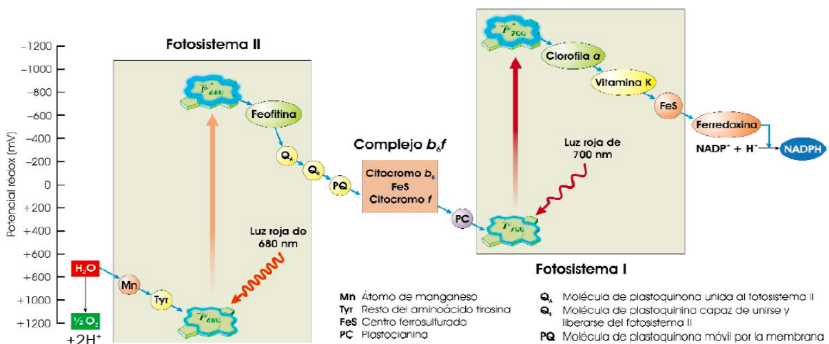
Ilustración 9.13. Puesta al día del diagrama de la ilustración 9.12. Suele denominarse esquema en Z porque, inicialmente, se representaba rotado 90° (hoy quizá sería más apropiado llamarlo “esquema en N”). (Fuente: ASH).
