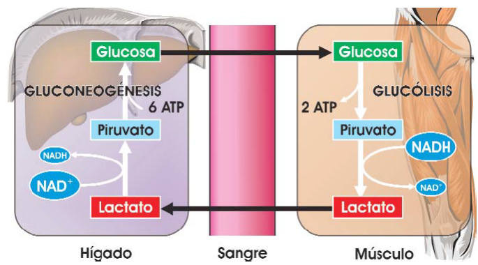
Ilustración 9.26. La diferente proporción NADH/NAD^+ en el músculo y en el hígado permite que el metabolismo de los azúcares discorra en sentidos opuestos (Fuente: ASH).
