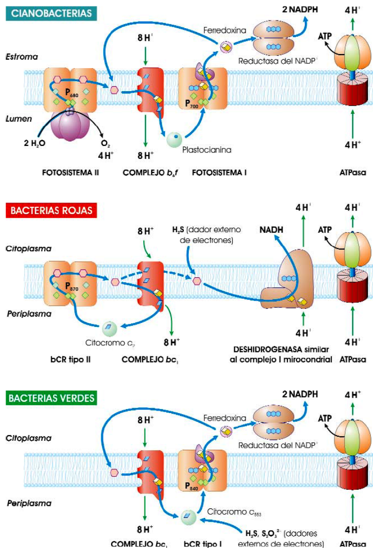
Ilustración 9.20. Comparación de la fotosíntesis de tres grupos de bacterias fotótrofas. Obsérvese que las bacterias rojas tienen un fotosistema (el centro de reacción bacteriano, o bCR) similar al PS II, mientras que el de las bacterias verdes recuerda al PS I (Fuente: ASH).
