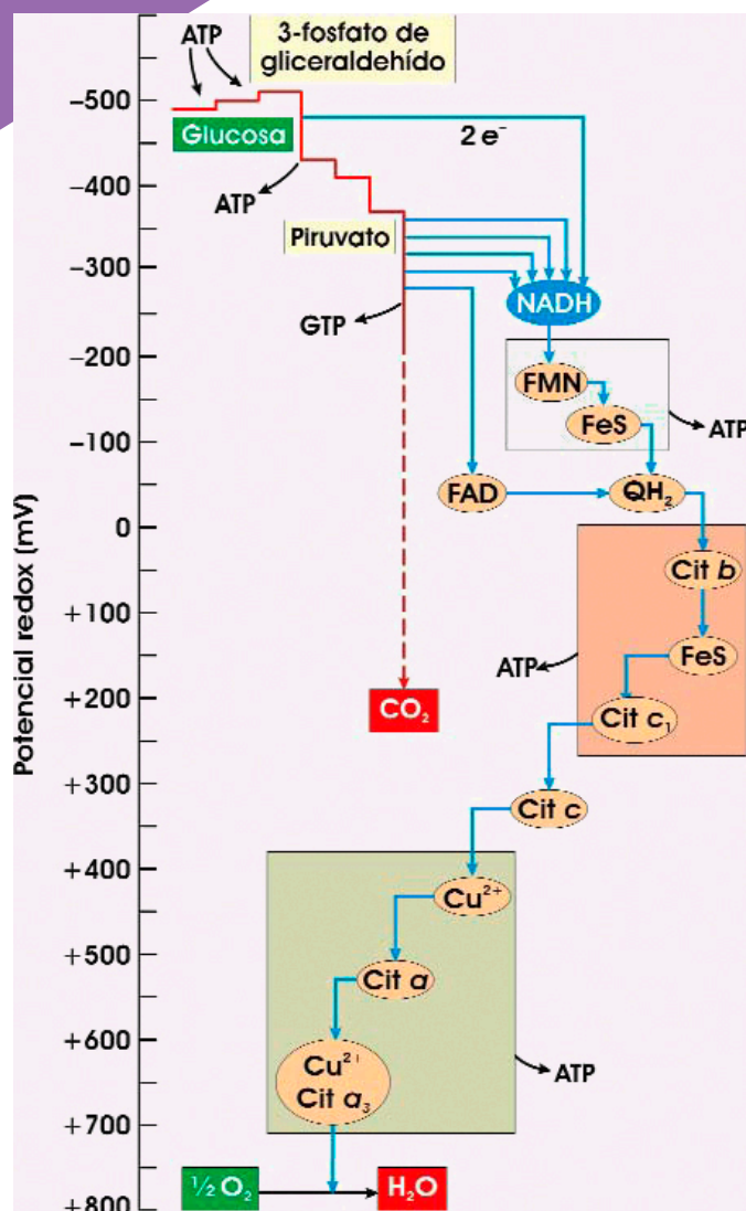
Ilustración 9.1. El flujo de electrones "escalera abajo" durante la respiración, desde la glucosa hasta el oxígeno (Fuente: ASH).
