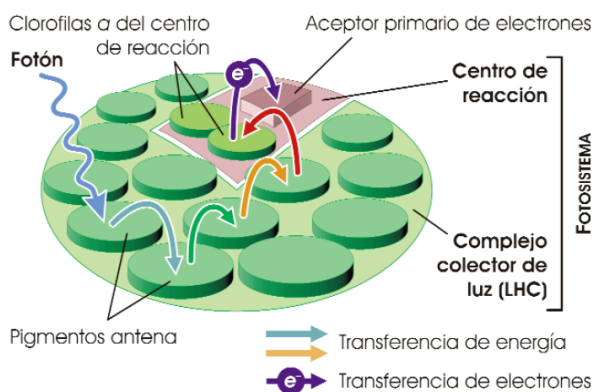
Ilustración 9.7. Estructura de un fotosistema. Obsérvese que la energía se transmite a través de pigmentos que absorben luz a longitudes de onda progresivamente mayores (Fuente: ASH).
