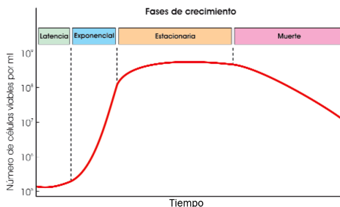
Ilustración 9.19. Curva de crecimiento de una bacteria. Fase de latencia: adaptación a las nuevas condiciones del medio. Fase exponencial o logarítmica: la velocidad de crecimiento es máxima y el tiempo de generación es mínimo. Fase estacionaria: se mantiene el número de bacterias. Fase de muerte: se produce una reducción del número de bacterias viables del cultivo. (Fuente: ASH).
