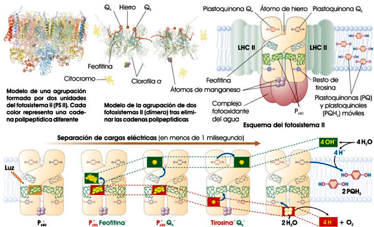
Ilustración 9.16. La transferencia secuencial de electrones, uno a uno, en el fotosistema II, induce una separación de cargas eléctricas positivas (recuadros rojos, abajo) y negativas (recuadros verdes). (Fuente: ASH).
