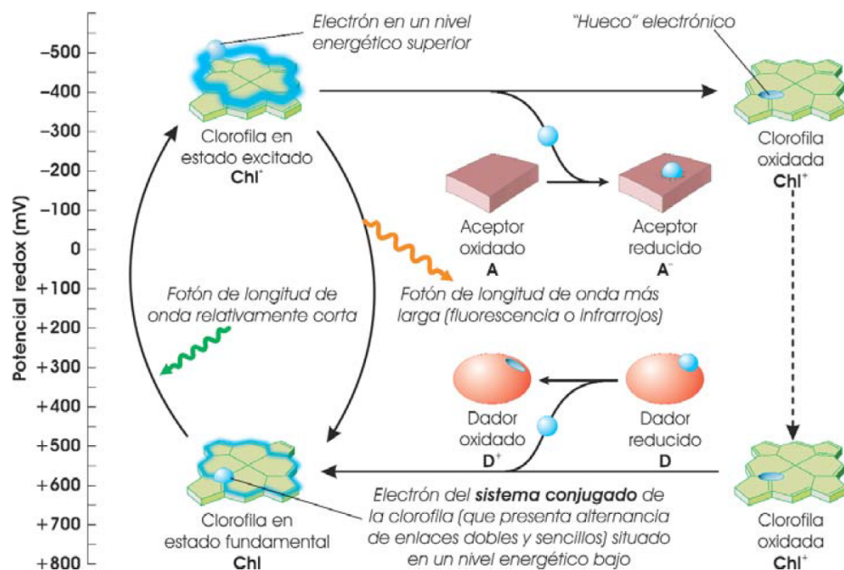
Ilustración 9.5. La clorofila tiene la extraordinaria propiedad de alternar entre dos potenciales redox distintos, interconvertibles gracias a la absorción o emisión de fotones. En el potencial bajo es capaz de ceder electrones a un aceptor adecuado, y en el alto puede tomarlos de un dador (Fuente: ASH).
