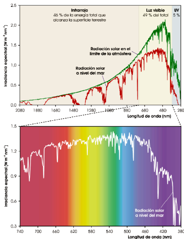
Ilustración 9.4. Irradiancia (cantidad de energía que llega a 1 m^2 de superficie en 1 s) de las distintas radiaciones electromagnéticas que inciden sobre la Tierra (Fuente: ASH).
