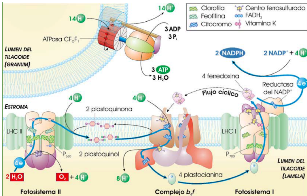
Ilustración 9.17. El flujo de electrones no cíclico desde el \text{H}_2\text{O} hasta el \text{NADP}^+ involucra a los fotosistemas I y II, pero en el flujo cíclico solo interviene el PS I. En ambos casos se bombean \text{H}^+ al lumen tilacoide, que luego servirán para la síntesis de ATP (Fuente: ASH).
