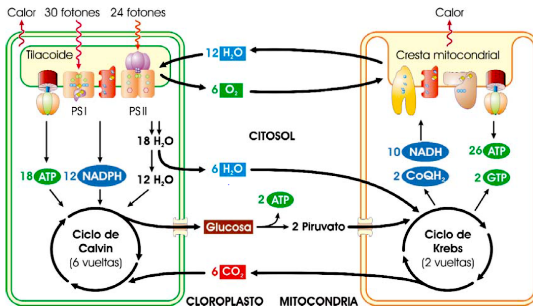
Ilustración 9.18. Esquema final del ciclo del carbono a nivel celular. Hay que advertir que, en realidad, la glucosa no es un producto del ciclo de Calvin. Aquí aparece simplemente por conveniencia, para posibilitar una comparación con la respiración celular, en la que la glucosa se oxida hasta CO_2 . Los productos del ciclo de Calvin son triosas fosfatadas, y los azúcares que se producen en las plantas son, principalmente, la sacarosa y el almidón, cuya síntesis ocurre sin pasar por una etapa de glucosa libre (Fuente: ASH).
