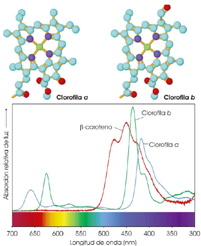
Ilustración 9.6. Espectros de absorción de las clorofilas a y b y del β-caroteno. Las diferencias de absorción entre los dos tipos de clorofila se deben únicamente a la sustitución de un grupo metilo por un aldehído (Fuente: ASH).
